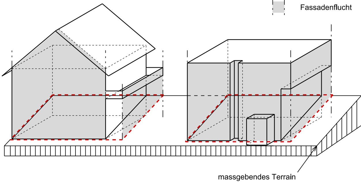
Figur 3.1 bis 3.3 Fassadenflucht und Fassadenlinie
