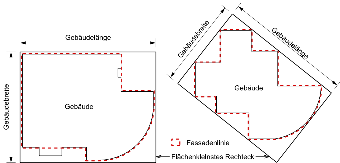
Figur 4.1 und 4.2 Gebäudelänge, Gebäudebreite
