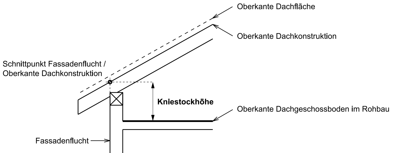
Figur 5.3 Kniestockhöhe
