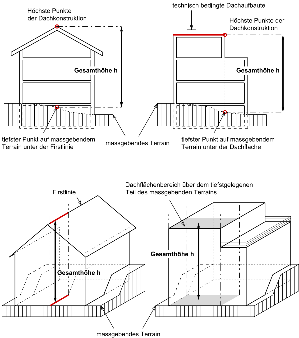
Figur 5.1 Gesamthöhe
