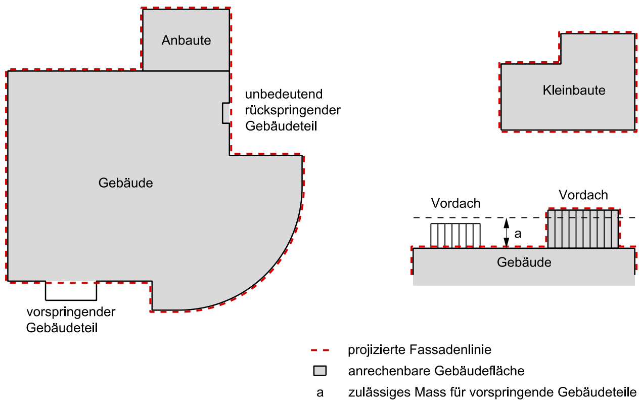
Figur 8.4 Anrechenbare Gebäudefläche
