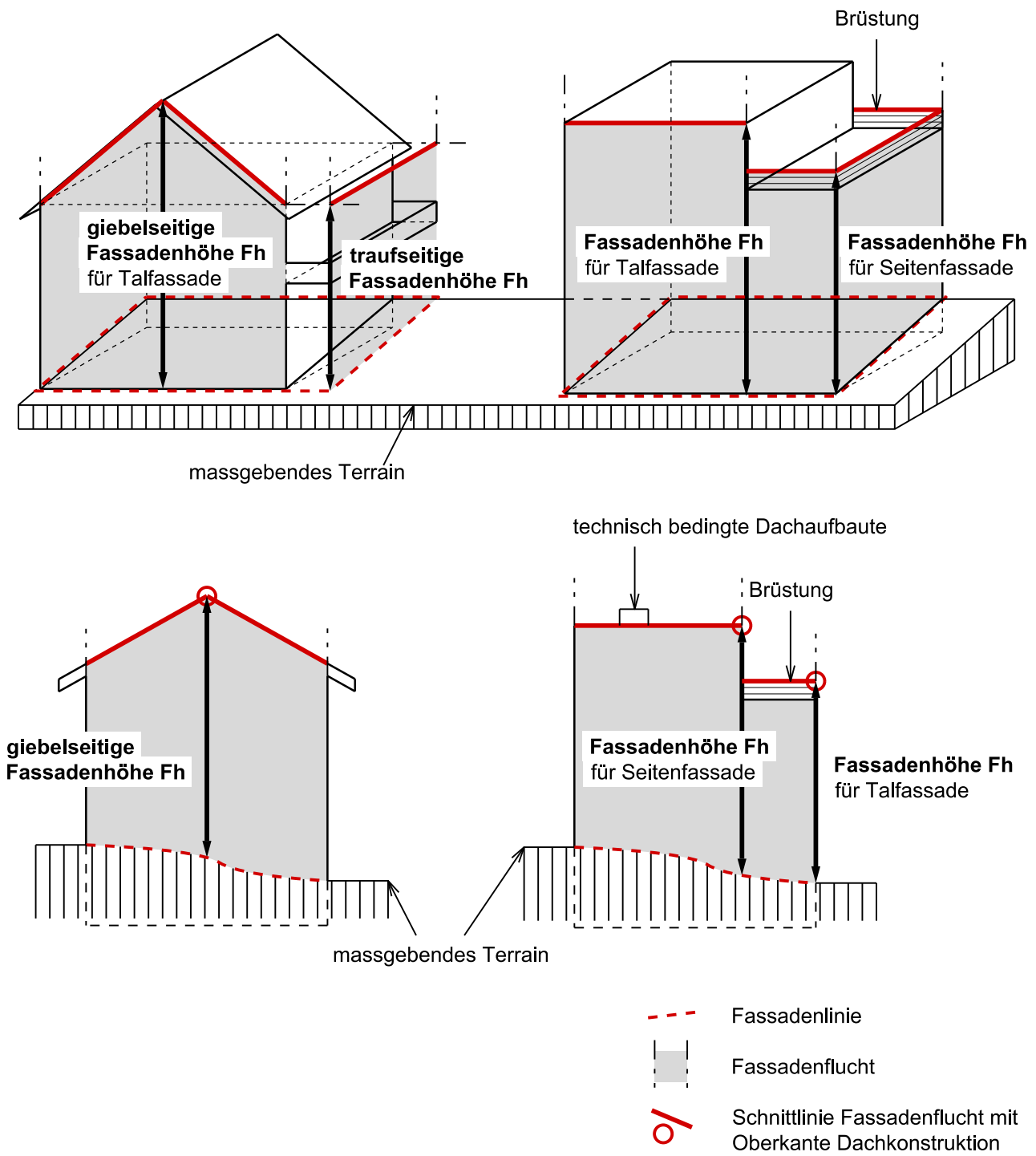
Figur 5.2 Fassadenhöhe
