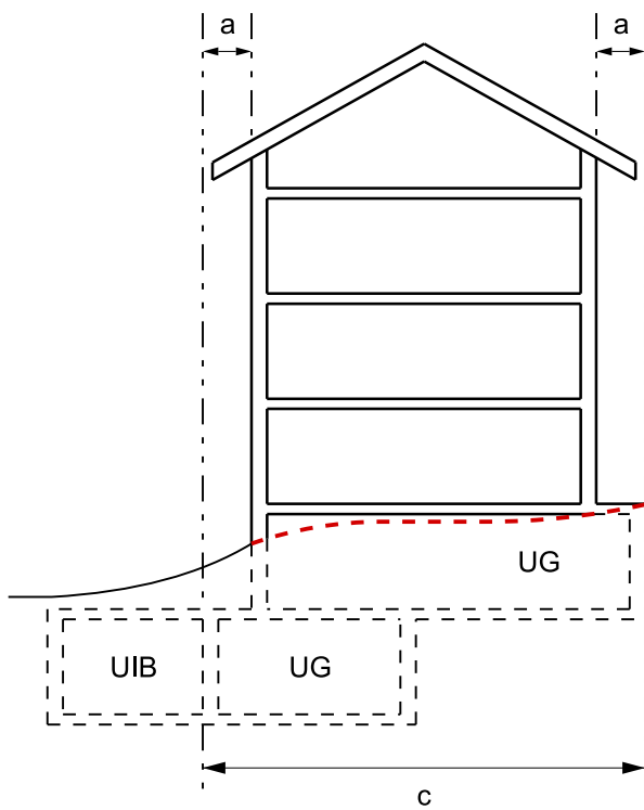
Figur 6.2 Untergeschosse
