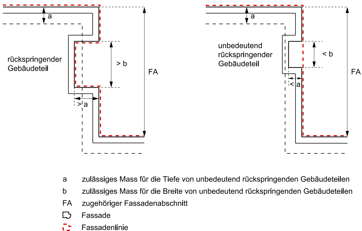
Figur 3.5 Rückspringende und unbedeutend rückspringende Gebäudeteile
