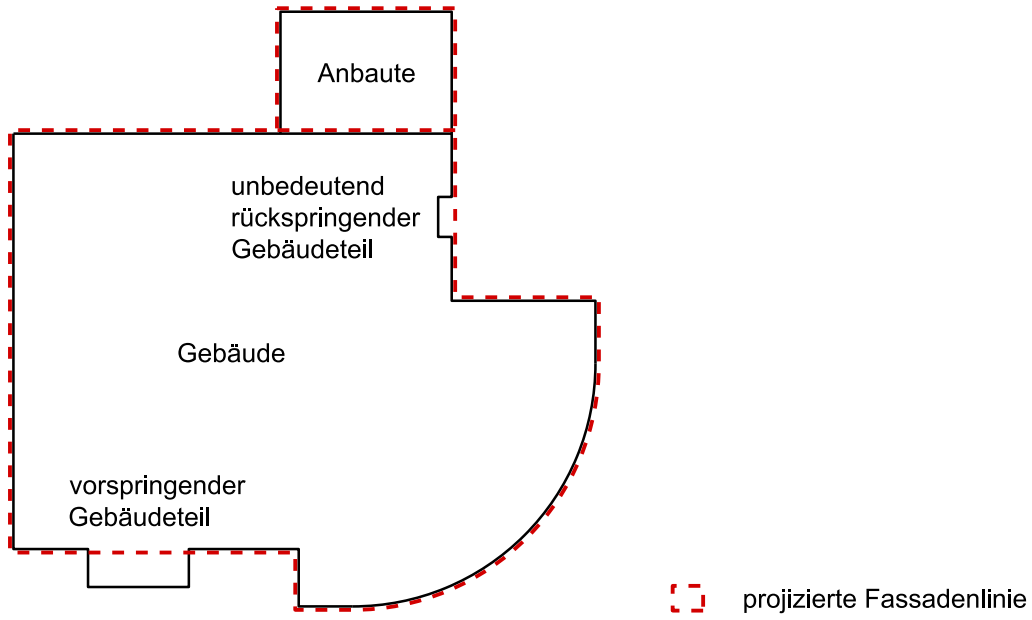
Figur 3.3 Projizierte Fassadenlinie
