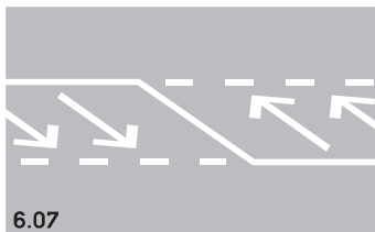
6.07 Abweispfeile (Art. 74)
