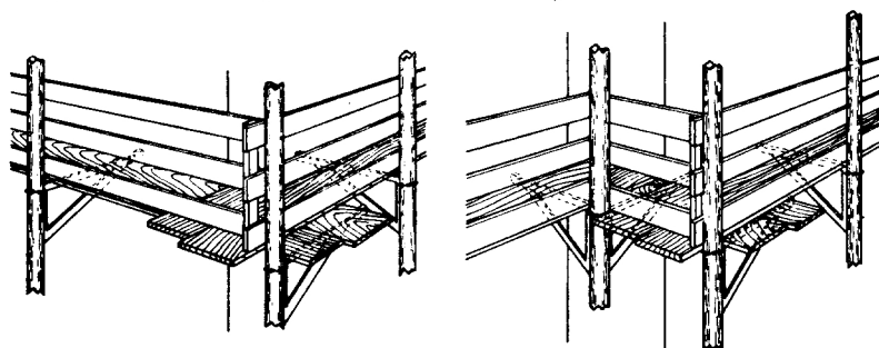
Extrémité et angles d'échafaudage
