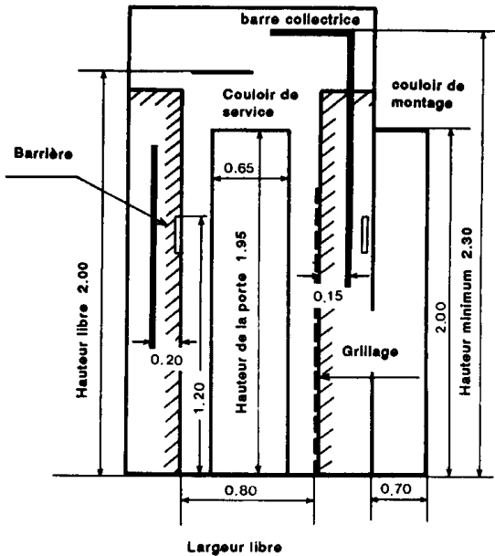
Distance minimale entre éléments sous tension et barrières, grillages ou panneaux pleins selon annexe 2 ch. 1
