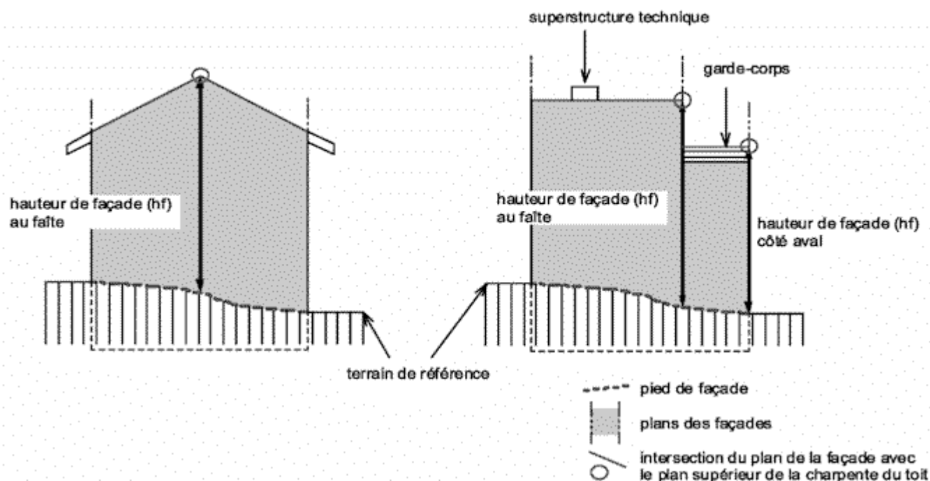
Figure 4.2.b Hauteur de façade
