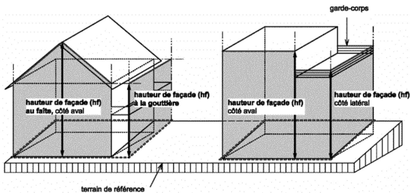
Figure 4.2.a Hauteur de façade
