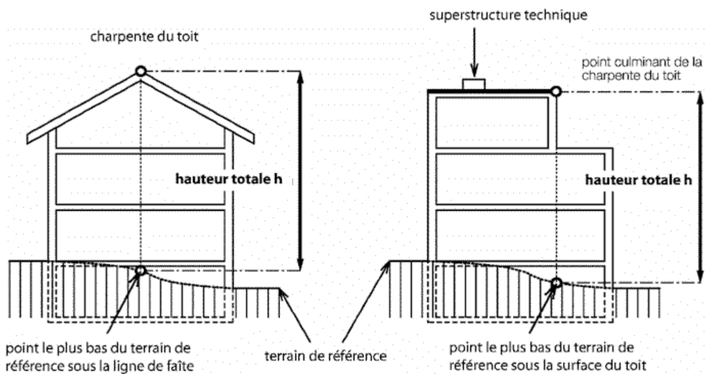
Figure 4.1.a Hauteur totale
