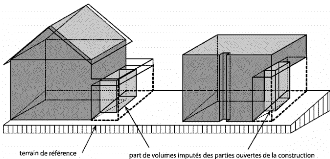
Figure 7.3 Indice de masse
