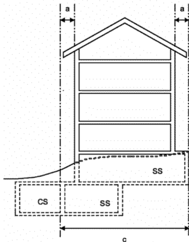
Figure 5.2 Sous-sols
