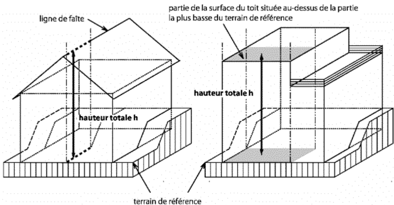
Figure 4.1.b Hauteur totale
