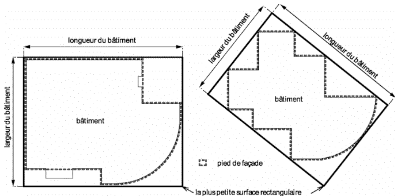
Figure 3.1 et 3.2 Longueur du bâtiment, largeur du bâtiment
