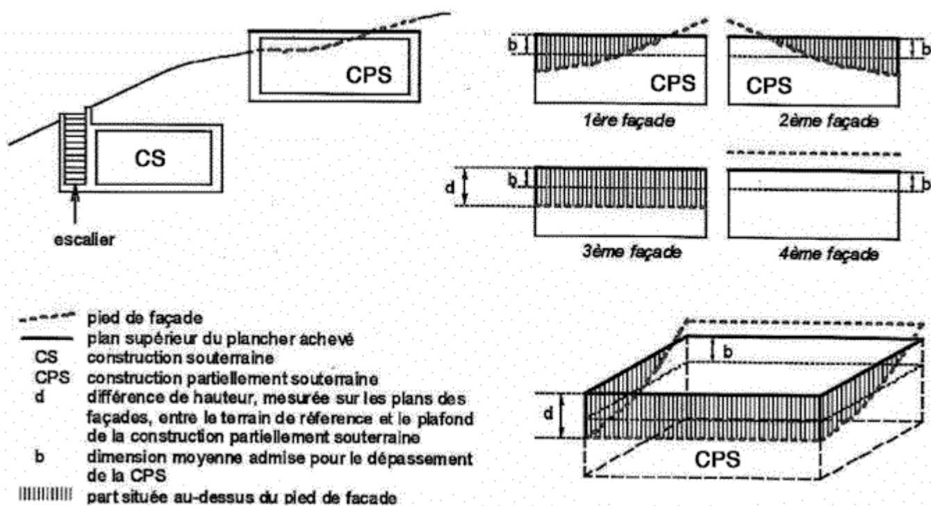
Figure 1.3 et 1.4 Constructions souterraines, constructions en sous-sol
