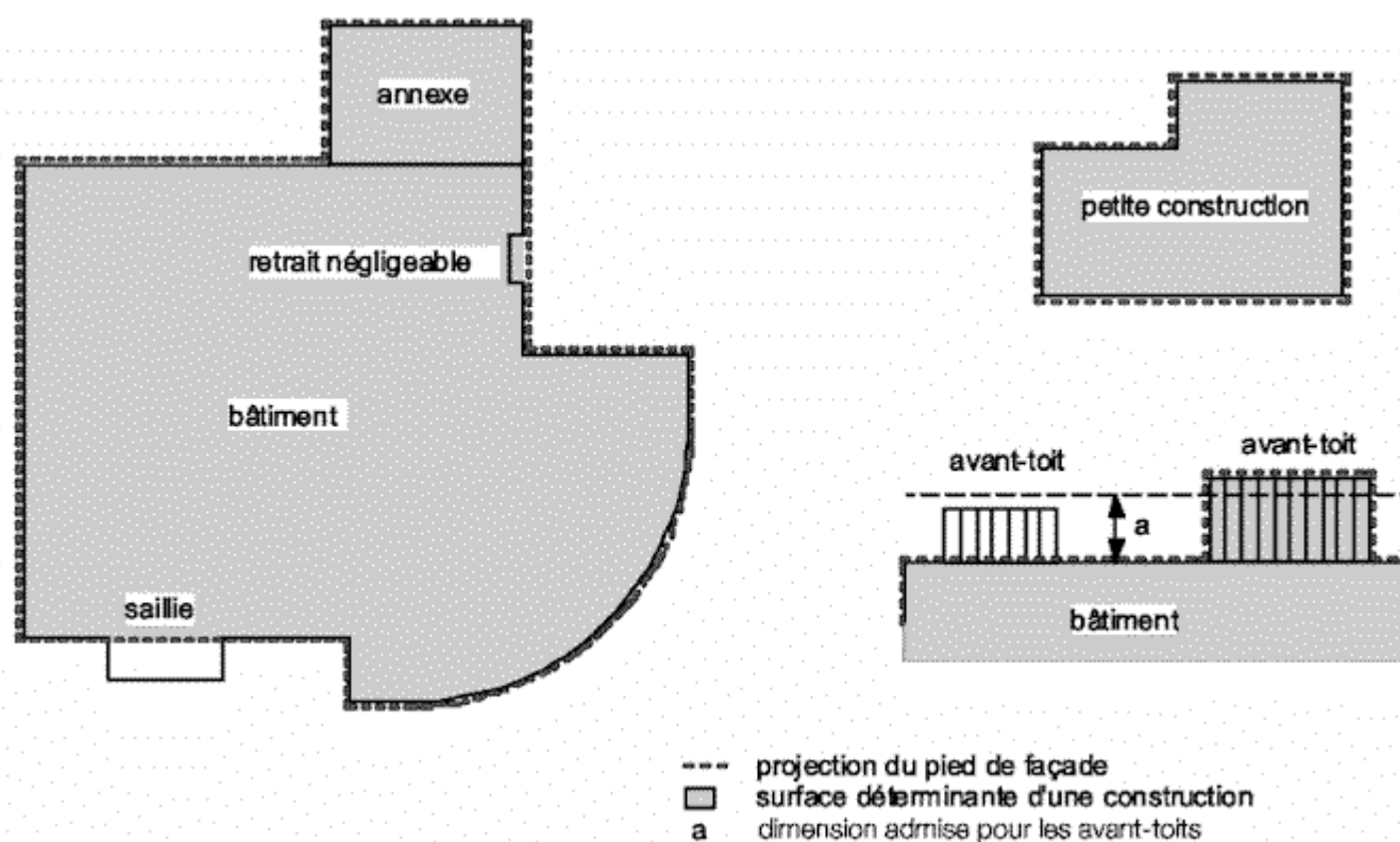
Figure 7.4 Surface déterminante d'une construction
