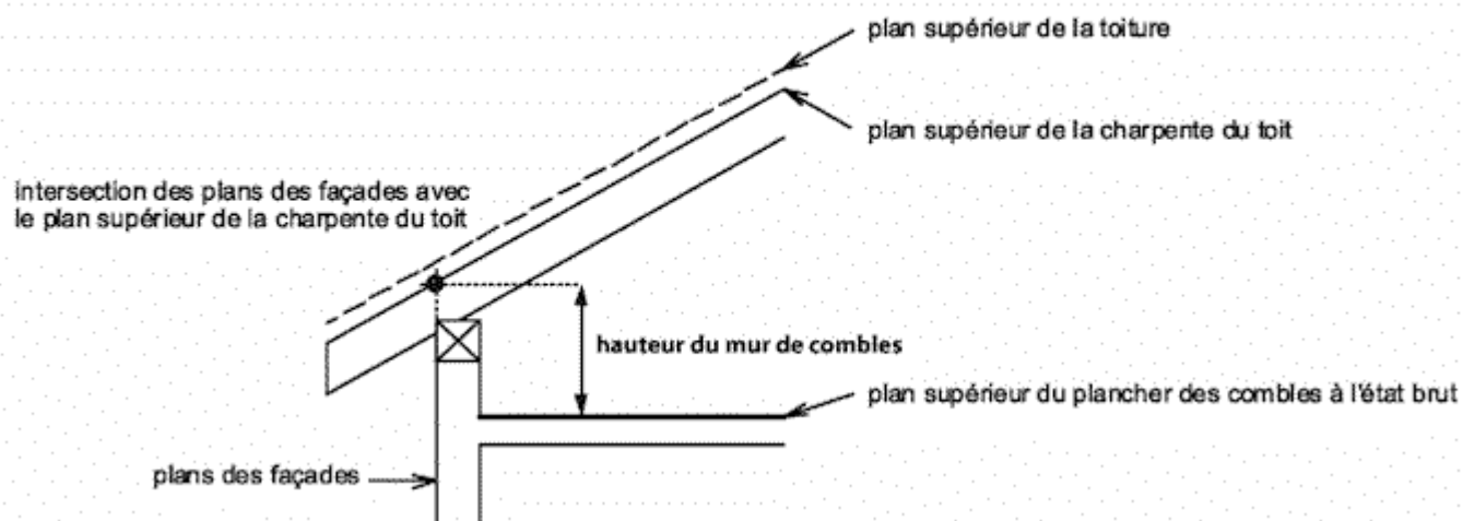
Figure 4.3 Hauteur du mur de combles
