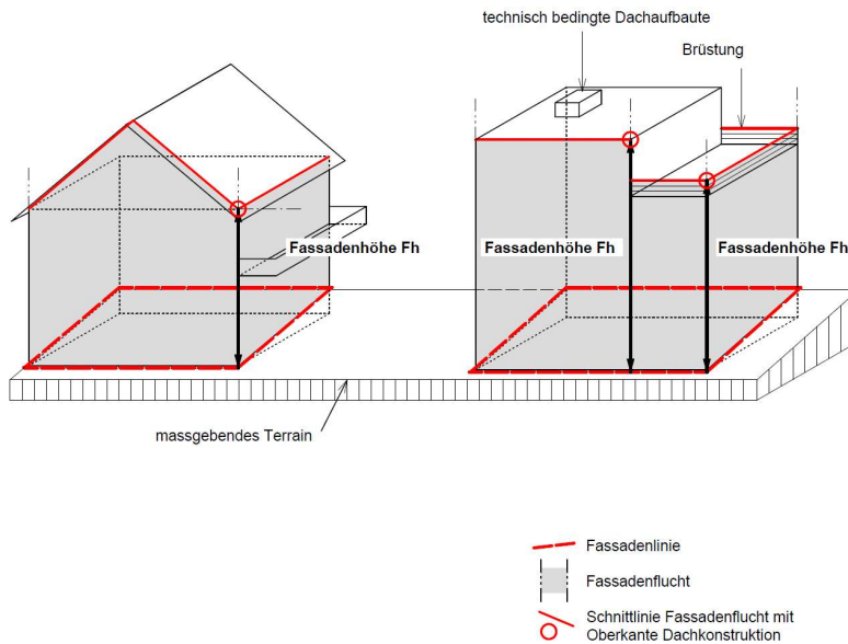
Figur 6 Fassadenhöhe
