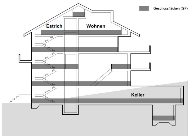
Schnitt:
