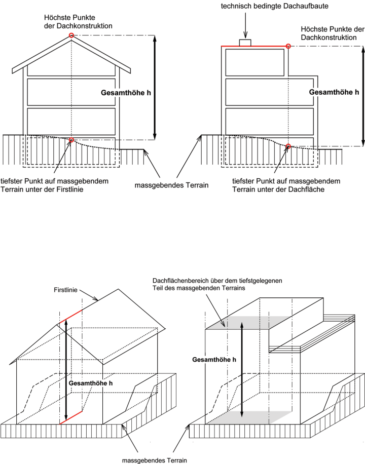
Figur 5.1 Gesamthöhe
