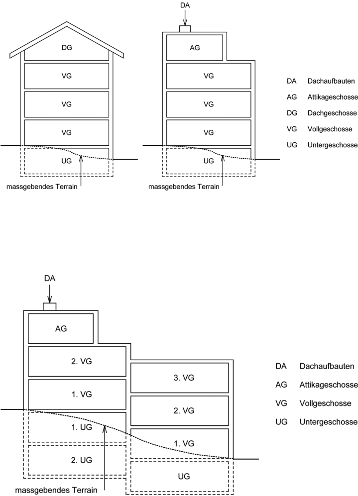
Figur 6.1 Geschosse und Geschosshzahl
