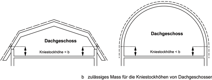
Figur 6.3 Dachgeschosse
