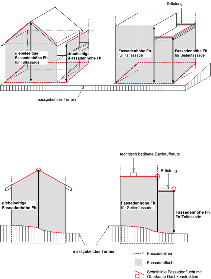
Figur 5.2 Fassadenhöhe
