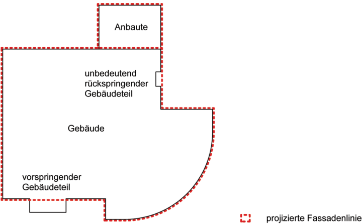
Figur 3.3 Projizierte Fassadenlinie
