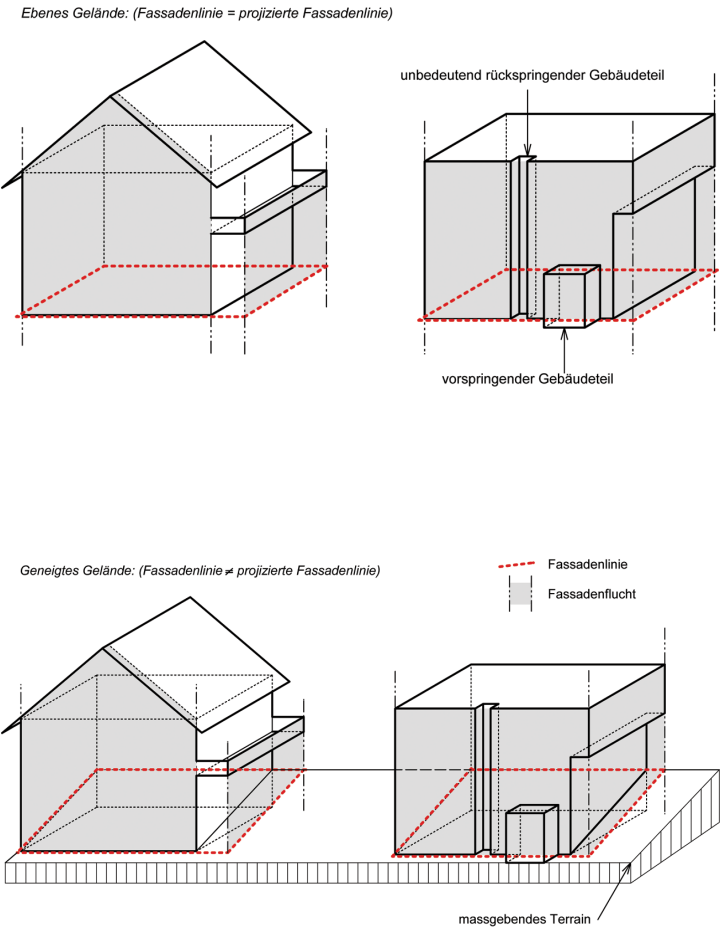
Figur 3.1 – 3.3 Fassadenflucht und Fassadenlinie
