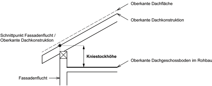
Figur 5.3 Kniestockhöhe
