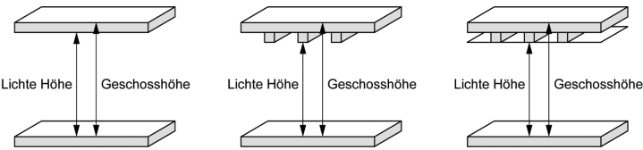
Figur 5.4 Lichte Höhe
